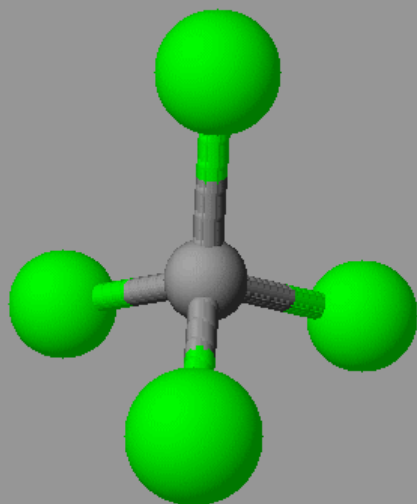
Tétrachlorométhane
