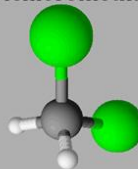
Dichlorométhane
