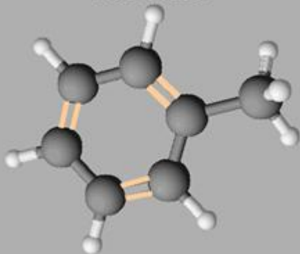
Toluène
