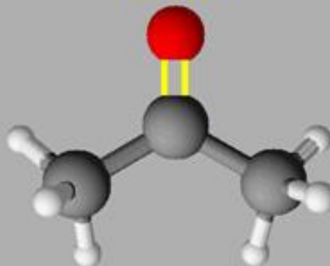
Acétone
